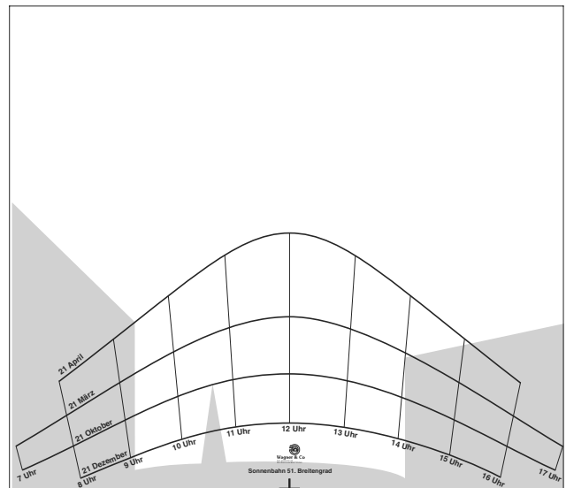
Bild 5 Die Gebäude und Baumrisse können Sie auf die Sonnenbahnfolie oder auf eine zweite dahintergeklebte Folie mittels wasserlöslichem Folienschreibers aufzeichnen. Den zukünftigen Standort der Solaranlage aufsuchen.
